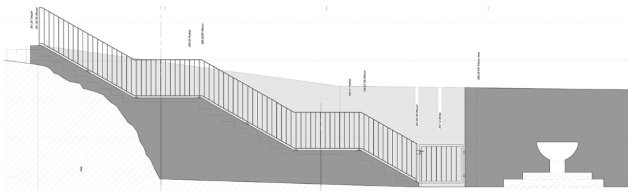
Detailplanung Trepenaufgang
